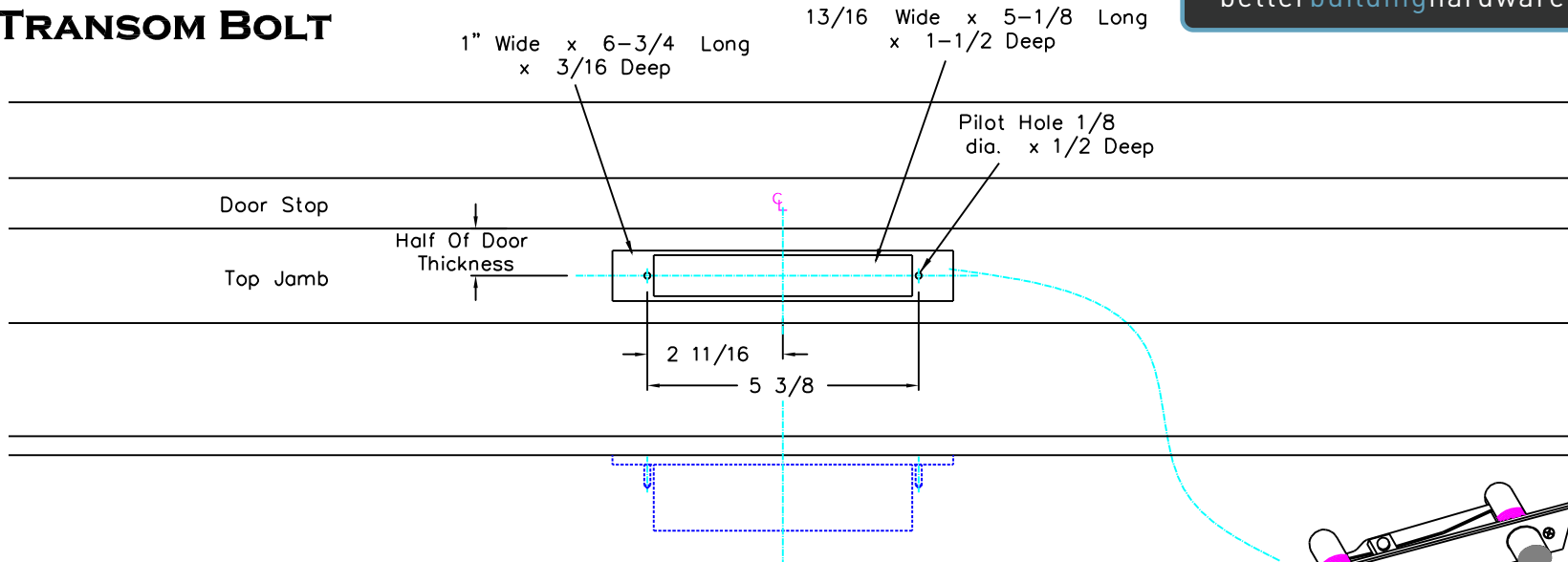
TRANSOM BOLT
